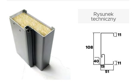
Ościeżnica "11" Protect
