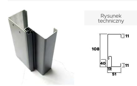
Ościeżnica "11" Premium / Normal
