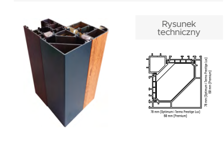
Przekrój łącznika kątownego Termo 90°
