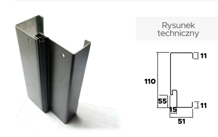
Ościeżnica "12" Optimum
