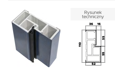
Ościeżnica aluminiowo-kompozytowa Optimum
