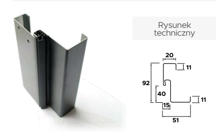
Ościeżnica "9" Premium / Normal
