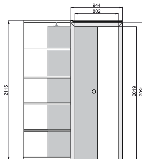
ÓŚCIEŻNICA ZAKRES 125 – STAŁY
