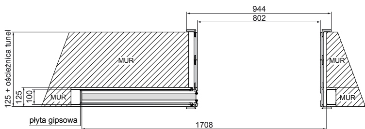
ÓŚCIEŻNICA ZAKRES (200-220) DO (400-420) – ASYMETRYCZNA
