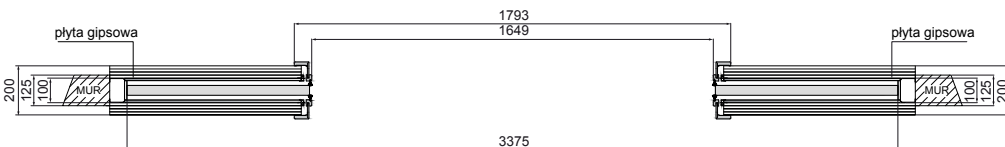
ÓŚCIEŻNICA ZAKRES (126-200) – SYMETRYCZNA*
