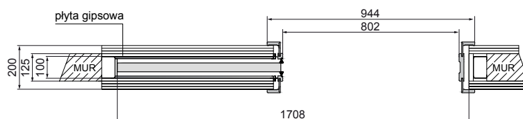
ÓŚCIEŻNICA ZAKRES (200-220) DO (400-420) – ASYMETRYCZNA
