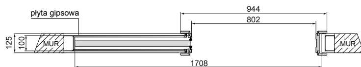
ÓŚCIEŻNICA ZAKRES (126-200) – SYMETRYCZNA*
